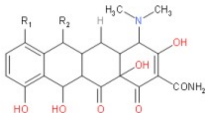
Gambar 7. Struktur tetrasiklin
