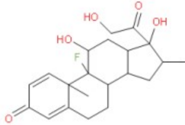
Gambar 5. Struktur deksametason
